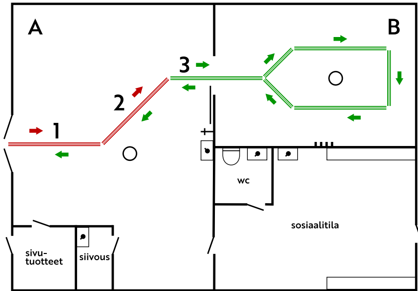
Yksinkertaisen lahtivajan periaate. Likaisen puolen toiminta punaisen ruhokiskon alueella, puhdas puoli vihreällä. Eläin tulee teurastilaan (A), asetetaan nylkypukille, piirretään ja vatsapuoli nyljetään (1). Eläin nyljetään loppuun ja nostetaan samalla riippumaan (2). Elinten poisto ja ruhon viimeistely kohdassa 3, josta ruho siirtyy jäähdytettyyn ruhovarastoon (B). Perusteellisen puhdistuksen jälkeen ruho voidaan palauttaa teurastilaan paloittelua ja leikkausta varten. (Lähde: Laaksonen, S. 2013. Metsästäjän terveysoppi, s. 247)
